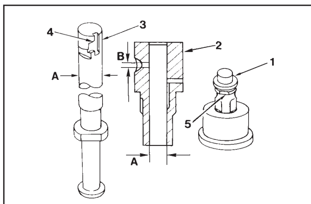
Elemento bomba y válvula de caudal para bomba inyección 6LD435 y 6LD435/V
