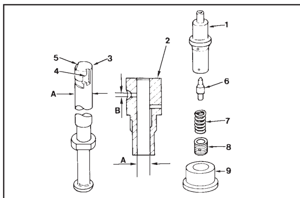
Elemento bomba y válvula de caudal GDV para bomba inyección 6LD401/B1 y 6LD435/B1
