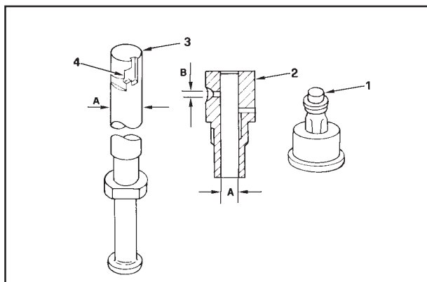
Elemento bomba y válvula de caudal para bomba inyección 6LD360, 6LD360/V, 6LD400 y 6LD400/V
